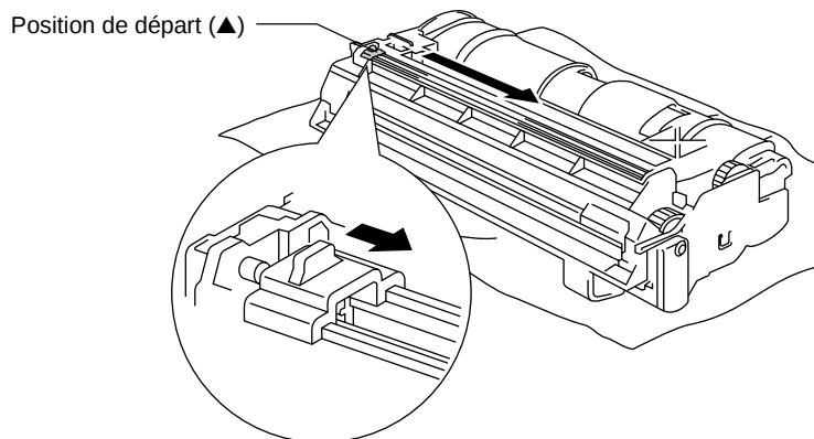
Fig. 5-9 Nettoyage du fil corona primaire
